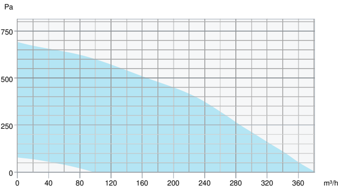
Abluft - Leistungskurve
