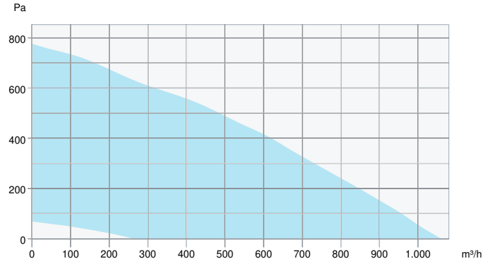
Abluft - Leistungskurve
