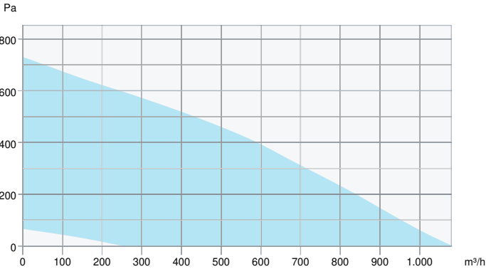
Zuluft - Leistungskurve
